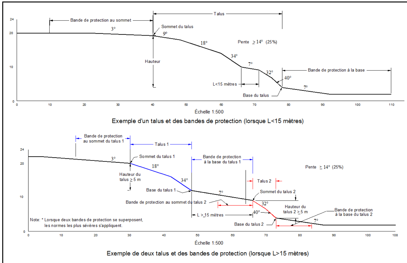
Figure 4 : Croquis d'un talus composé de sols à prédominance argileuse avec un plateau de moins de 15 m (croquis supérieur) et d'un plus de 15 m (croquis inférieur)
